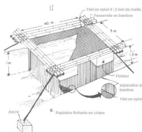
Conception d'un hapa flottant avec des poteaux ou des tonneaux sur la surface de l'étang
