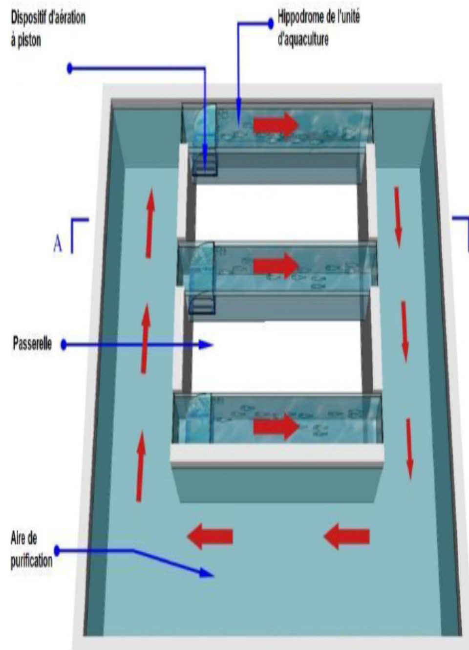
Conception schématique d'un IPRS avec un dispositif d'aération à bouchon pour le contrôle du débit et de la qualité de l'eau (Crédit: Li et al. 2019)
