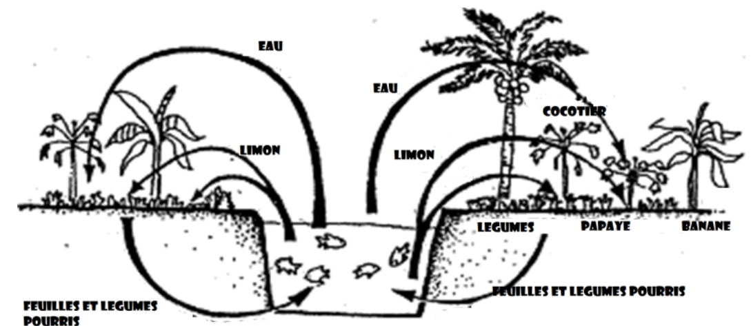
Concept de production intégrée de poissons et de cultures (Crédit: FAO)
