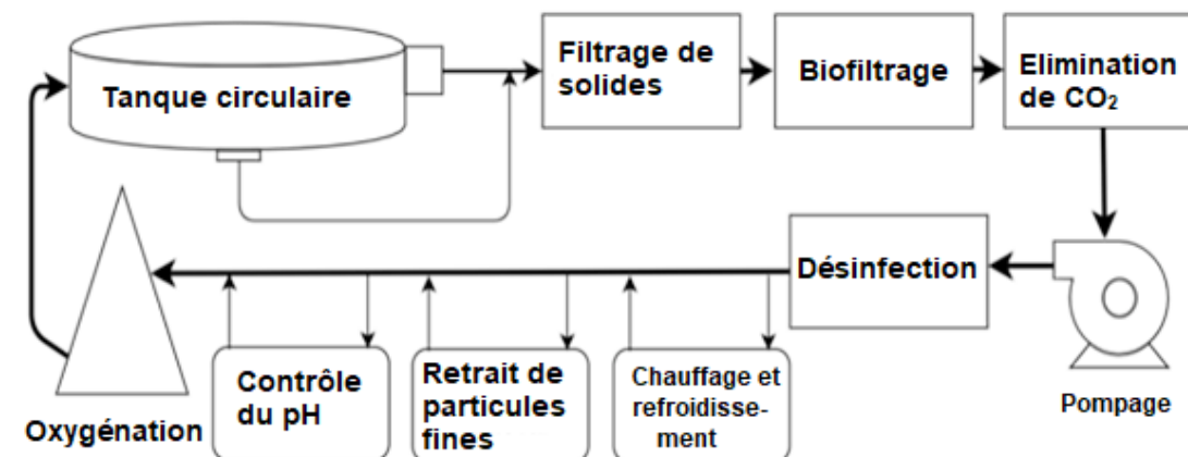
Conception schématique d'un système de recirculation
