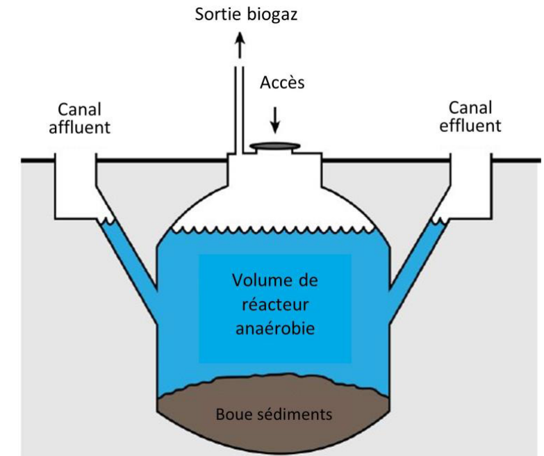
Schéma d'un réacteur anaérobie souterrain produisant du biogaz à partir de déchets agricoles
